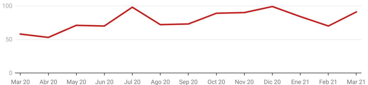
Figura 1: Ataques marzo 2020-21.
